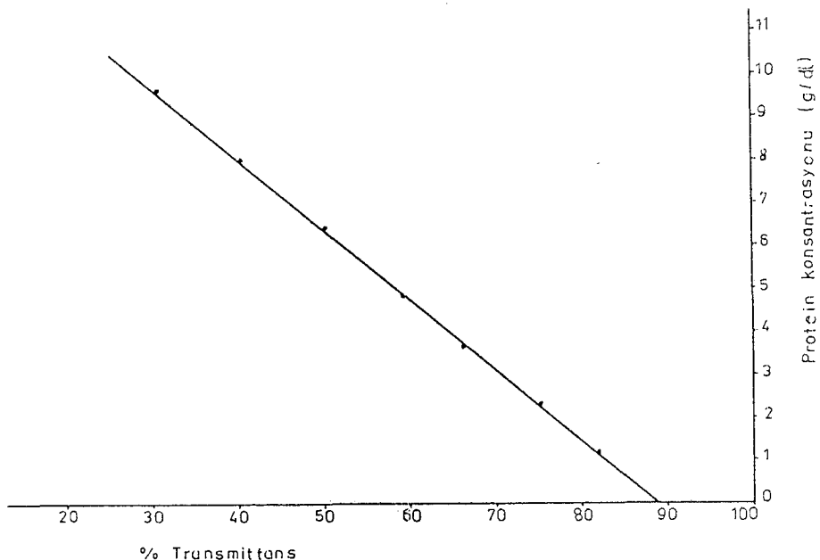
Şekil 3.4. T. protein standartına göre çizilen kalibrasyon eğrisi.
