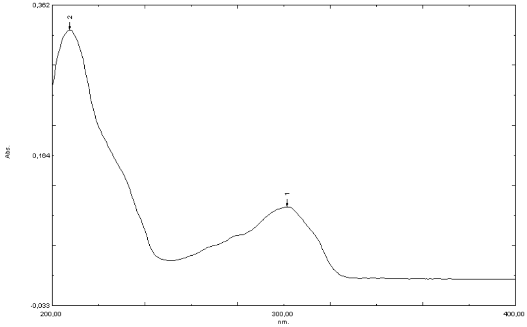
Şekil 5.2. Metanolde çözülmüş GRA'nın 200-400 nm arasında elde edilmiş spektrumu
