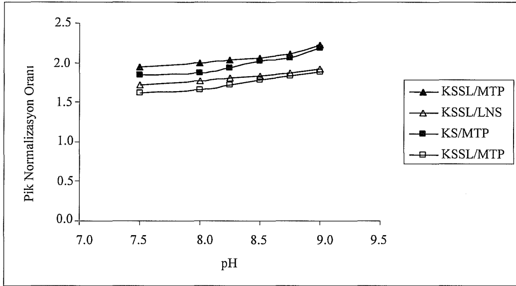
Şekil 25. pH'in Maddelerin Pik Normalizasyon Oranı Üzerine Etkilerinin Grafikselleştirilmesi
