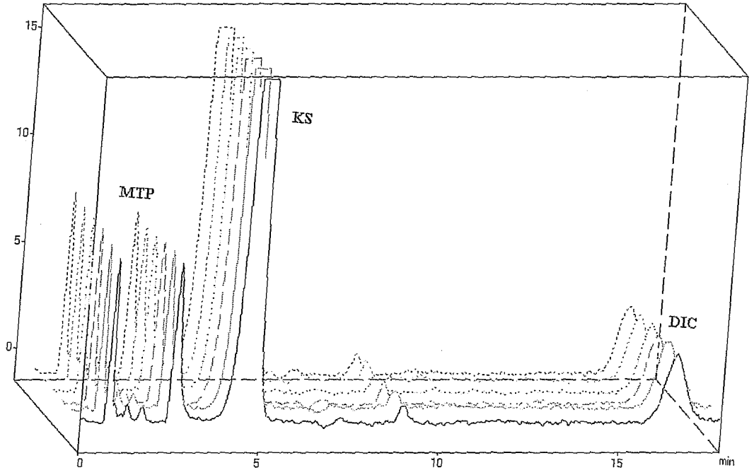
Şekil 45. Yüksek Performanslı Sıvı Kromatografisi Yönteminin Gün İçi Kesinliğinin Grafıksel Gösterimi 3 gün süresince yapılan toplam 18 enjeksiyona ait istatistiksel değerlendirmeler Çizelge 33'te sunulmaktadır.
