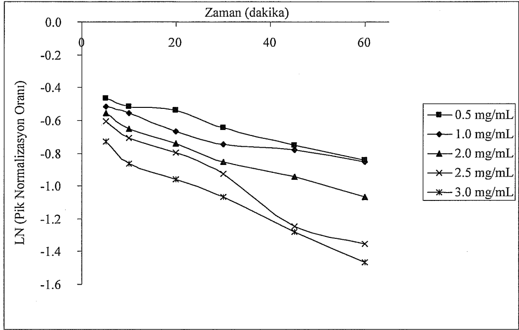
Şekil 51. Kapiler Elektrozef Yöntemi ile Mikrozoimal Protein Derişimi Analiz Sonularının Logaritmik Grafiđi
