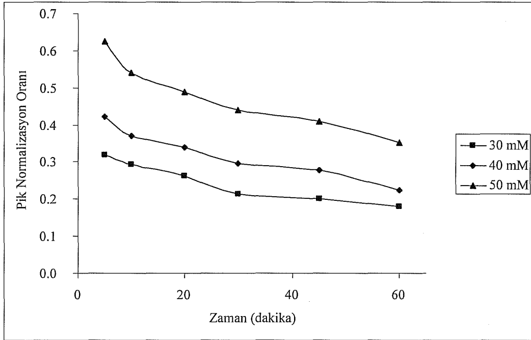
Şekil 52. Kapiler Elektrofrez Yöntemi ile Substrat Derişimi (Diklofenak Sodyum) Analizinin Grafikselsel Gösterimi
