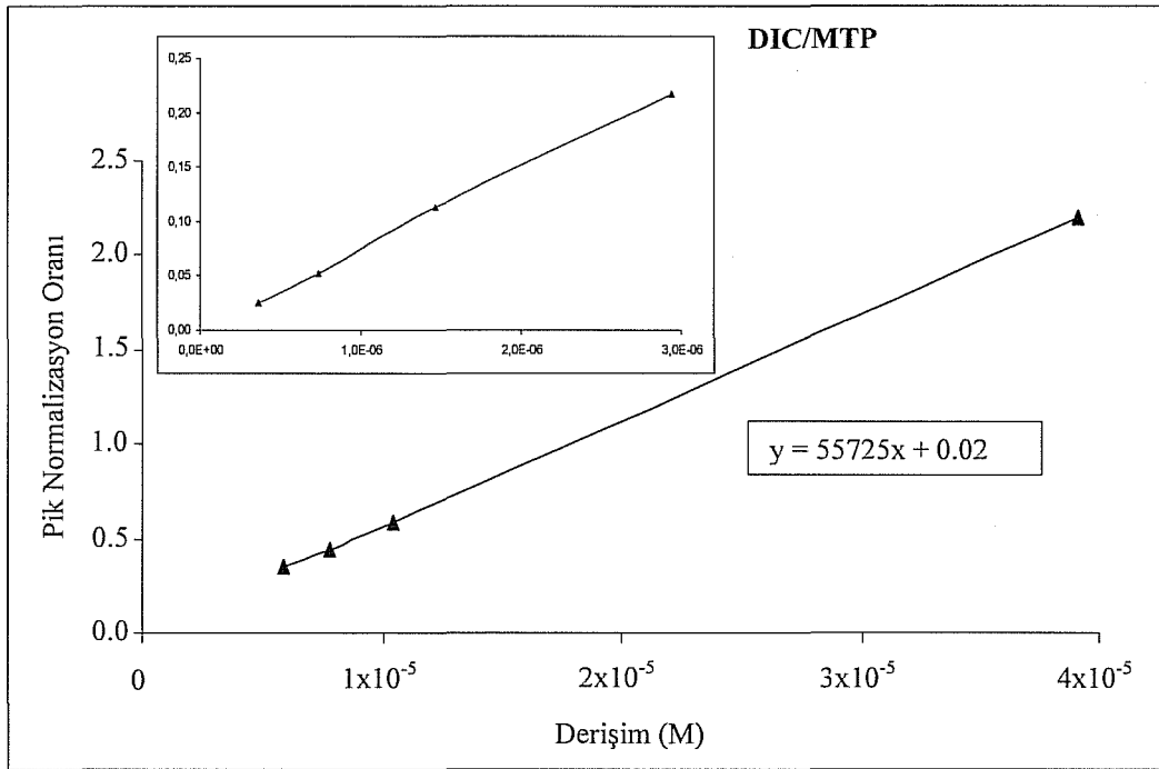
Şekil 43. Yüksek Performanslı Sıvı Kromatografisi Yönteminin Diklofenak Sodyum İçin Doğrusallığının Grafıksel Gösterimi
