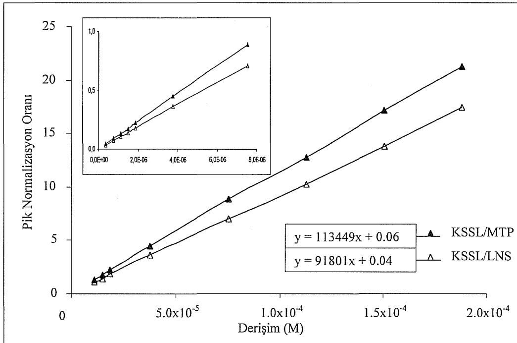
Şekil 37. Kapiler Elektroferez Yönteminin Kandesartan Sileksetil İçin Doğrusallığının Grafikselleştirilmesi
