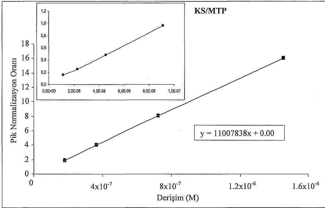
Şekil 42. Yüksek Performanslı Sıvı Kromatografisi Yönteminin Kandesartan İçin Doğrusallığının Grafıksel Gösterimi
