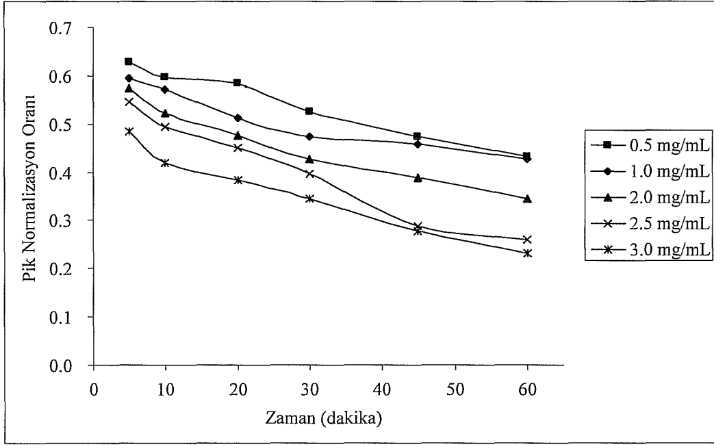
Şekil 50. Kapiler Elektroforez Yöntemi ile Mikrozomal Protein Derişimi Analizinin Grafiksel Gösterimi
