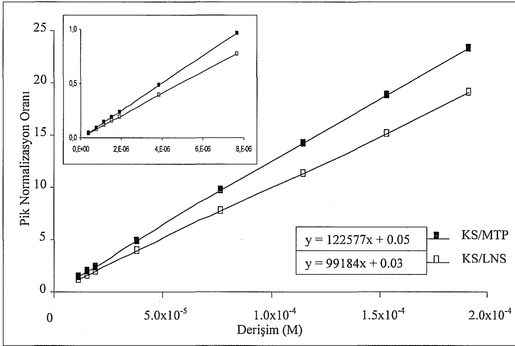
Şekil 36. Kapiler Elektroferez Yönteminin Kandesartan İçin Doğrusallığının Grafikselleştirilmesi
