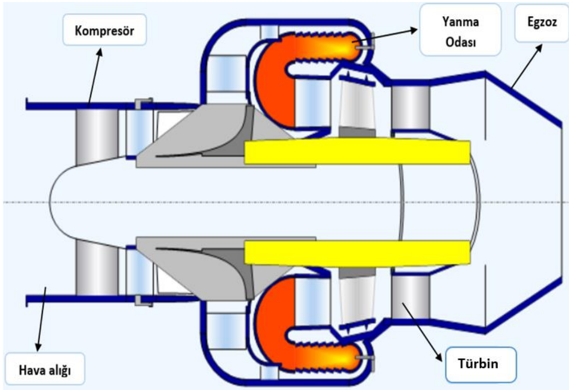
Şekil 3.1. TRS18 Turbojet motorunun tasarım şeması
