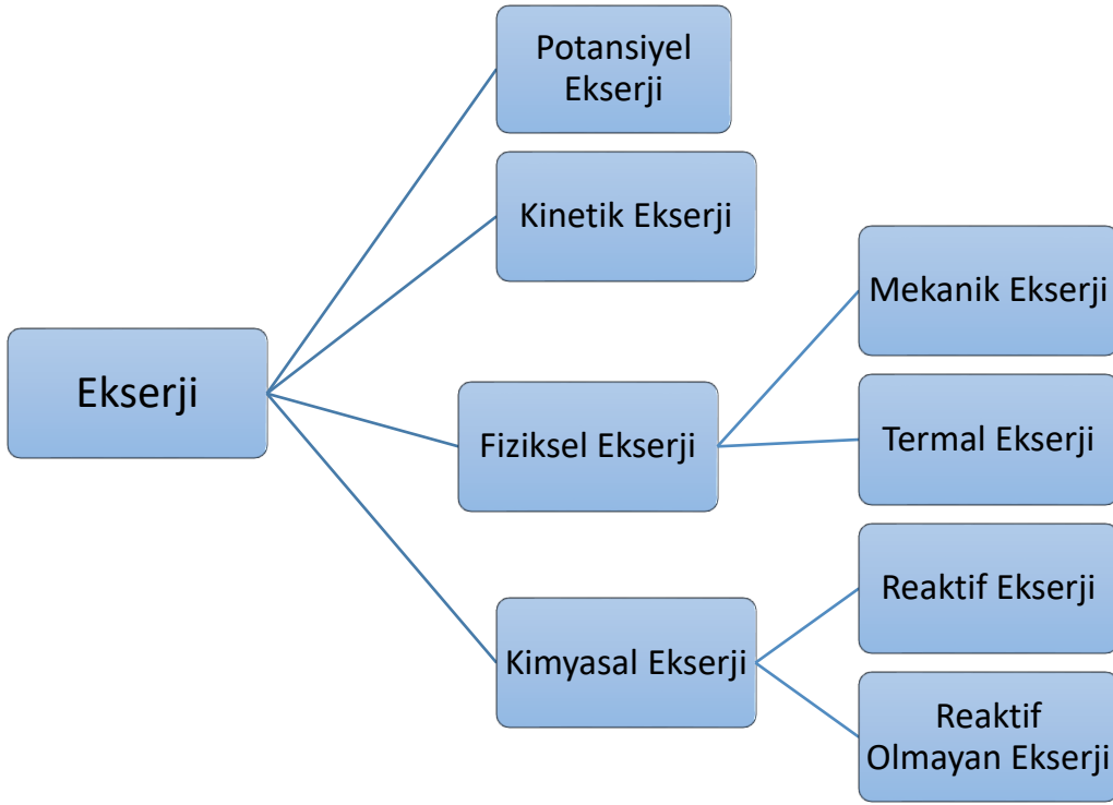
Şekil 4.1. Ekserji bileşenleri [26]
