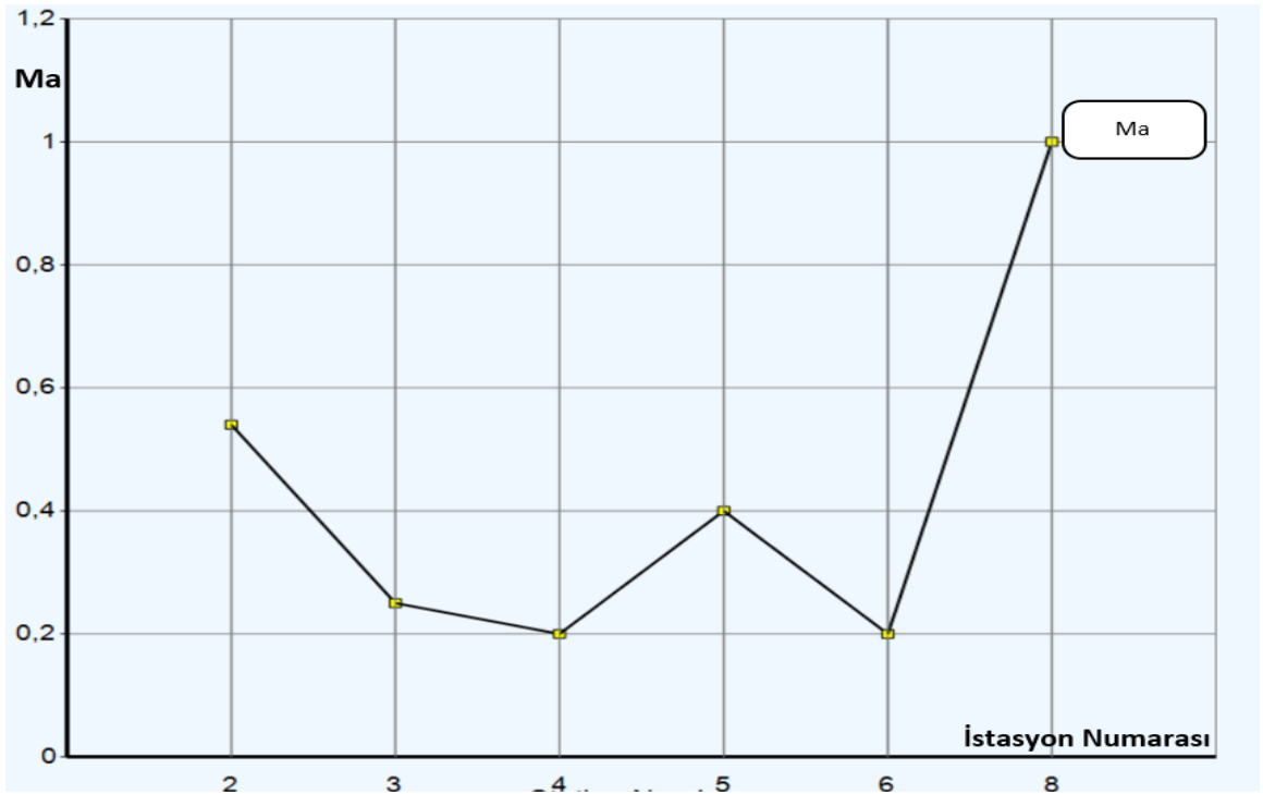
Şekil 5.8. TRS18 motoru Mach sayısı grafiği
