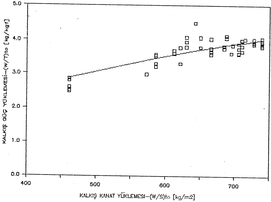
Şekil 3.3. W_{to} > 235000 kg. ağırlık grubu için (W/S)_{to} - (W/T)_{to} arasındaki pratik ve teorik ilişkiler.
