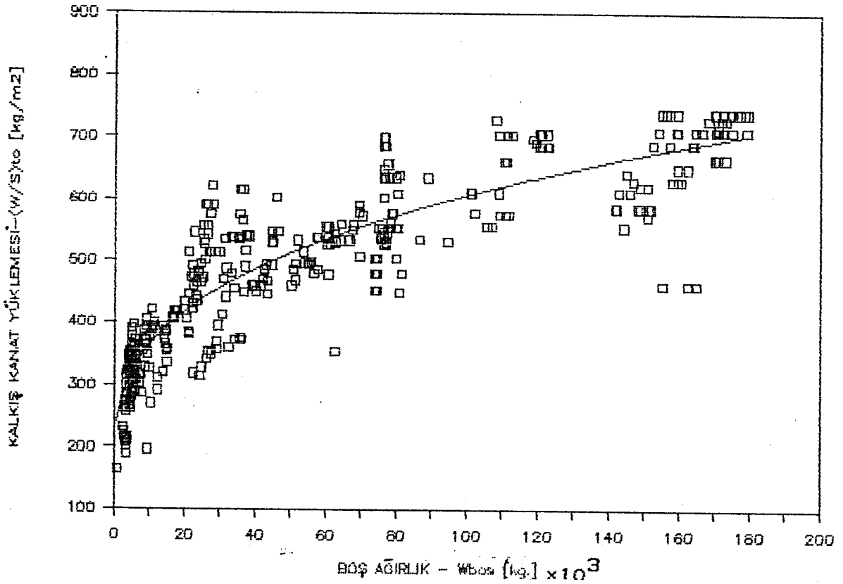
Şekil 6.1 Bütün uçaklar için boş ağırlık ve kalkış kanat yüklemesi arasındaki pratik ve teorik ilişkiler
