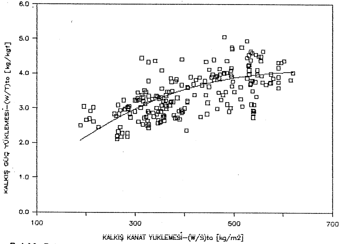
Şekil 3.7. W_{to} < 166000\text{kg} . (dar gövdeli) ağırlık grubu için (W/S)_{to} - (W/T)_{to} arasındaki pratik ve teorik ilişkiler.
