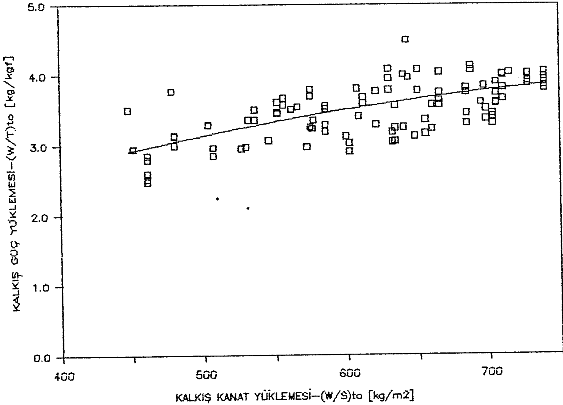
Şekil 3.6. W_{to} > 127000 kg. (geniş gövdeli) ağırlık grubu için (W/S)_{to} - (W/T)_{to} arasındaki pratik ve teorik ilişkiler.
