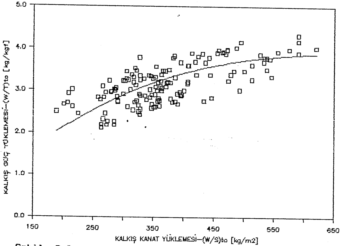
Şekil 3.4. W_{to} < 65000 kg. ağırlık grubu için (W/S)_{to} - (W/T)_{to} arasındaki pratik ve teorik ilişkiler.
