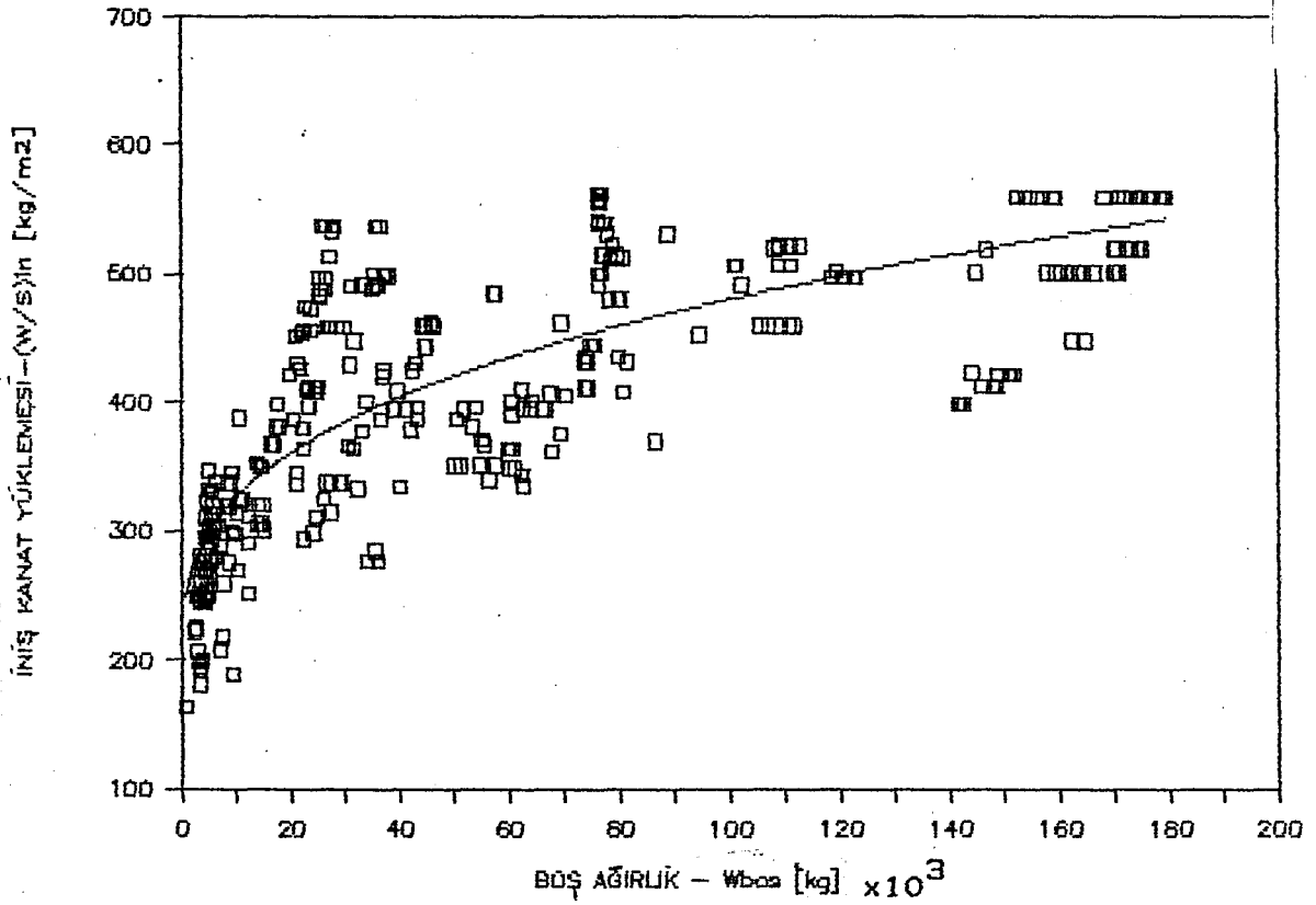
Şekil 6.4 Bütün uçaklar için boş ağırlık ve iniş kanat yüklemesi arasındaki pratik ve teorik ilişkiler
