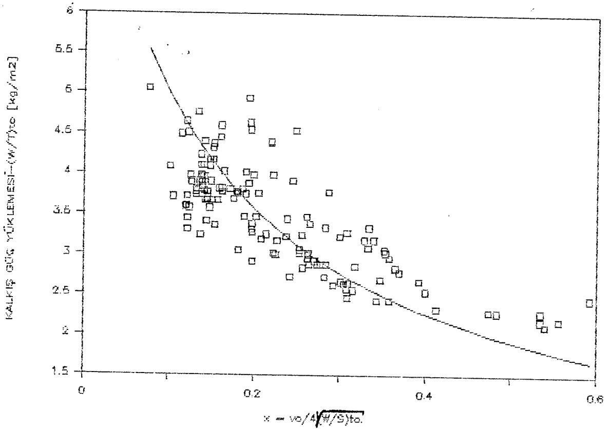
Şekil 5.2 (W/T)_{to} - v_o/4\sqrt{(W/S)_{to}} arasındaki teorik ve pratik ilişkiler.
