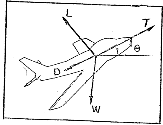
Şekil 5.1 Tırmanma hareketinde uçağa etki eden kuvvetler,
