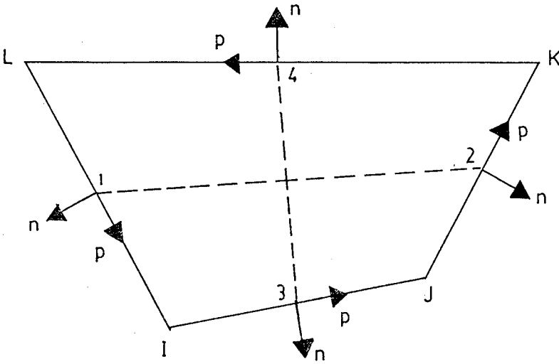
Şekil 5.5 Gerilme çıktılarının pozitif yönleri.
