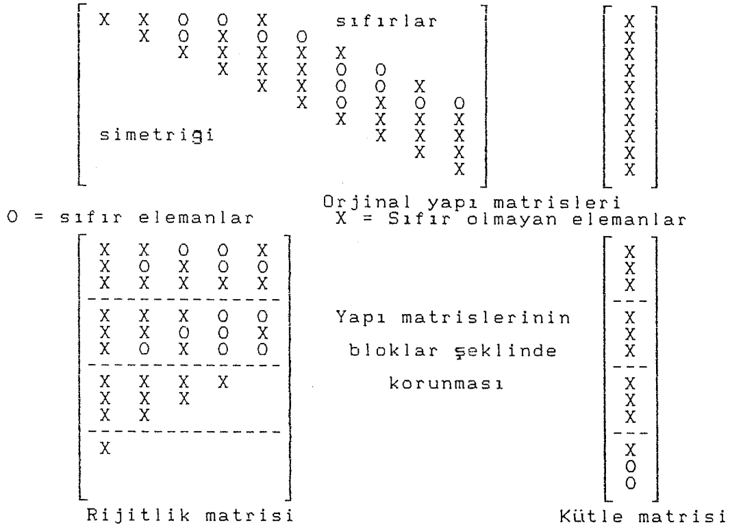
Şekil 4,4 Rijitlik ve kütle matrisinin bellekte korunması
