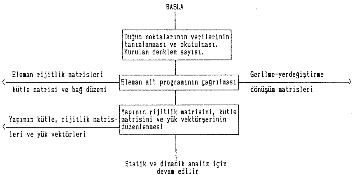
Şekil 4,5 Yapının kütle ve rijitlik matris hesapları için akış diyagramı.
