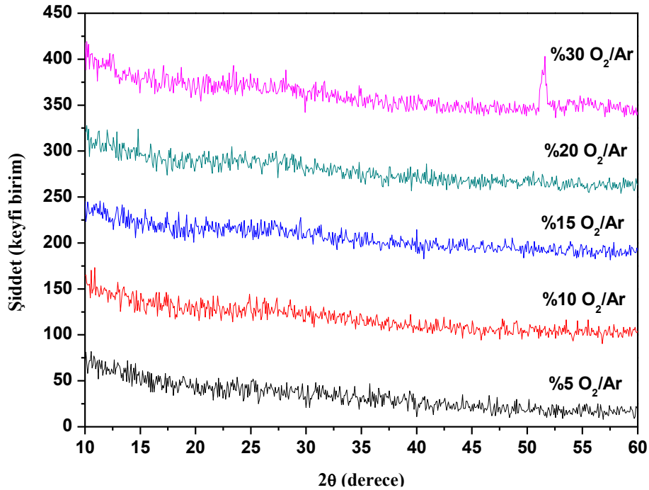
řekil 7.6. Si/SiN alttař üzerine 20 nm kalınlıkta 4 sccm argon gaz akıř ve % 5, 10, 15, 20 ve 30 O 2 /Ar gaz oranlarında üretilen VOx ince filmlerin GIXRD kırınımı desenleri. % 30 O 2 /Ar kırınım deseninde 53° derecede görölen pik XRD optik sisteminden kaynaklanan bir anomalidir, bir kristal yapıya ait deđildir.
