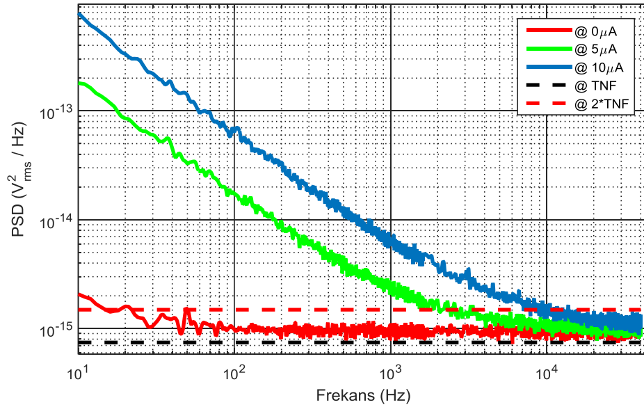
Şekil. 7.62: 200 °C'de 3 saat ısıl işlem gören VOx ince filmin 5, 10 μA akımlarında 1/f gürültüsü ölçüm grafikleri
