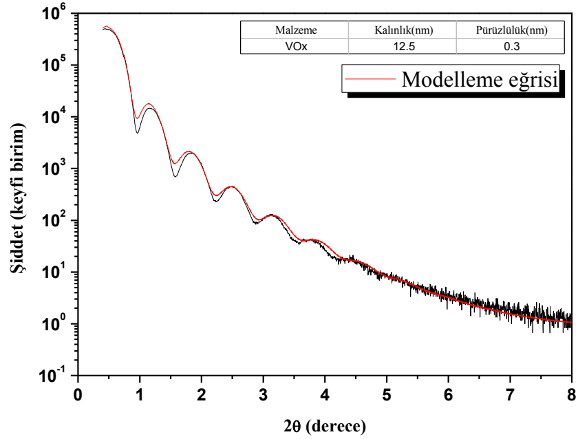
Şekil 7.1. 4/0.2 sccm Ar/O 2 gaz akış oranında üretilen numunenin XRR modelleme ve ölçüm eğrileri
