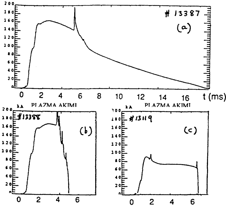
Şekil 7.3. Plazma akımı dalga formları: (a) hafif arttırılan dikey alan ( B_v ), (b) orta derecede arttırılan B_v , (c) büyük miktarda arttırılan B_v . [26]
