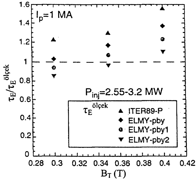
Şekil 7.18. Toroidal alanın bir fonksiyonu olarak dört ölçek değerine normalize edilmiş iki kaynaklı 1MA'lık boşalmalar için kuşatma zamanı [30]
