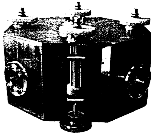
Şekil 7.20. Türkiye'de geliştirilen küresel tokamak modelinin akı koruyucusu [10]
