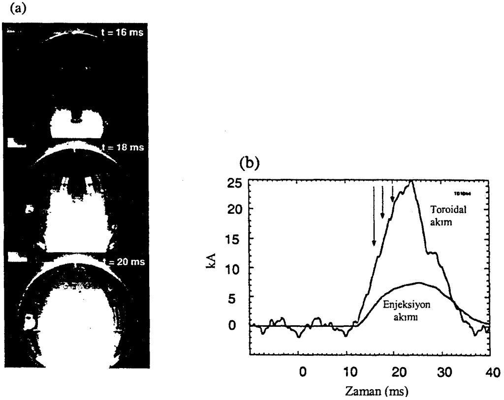
Şekil 7.17. (a) Hızlı kamera görüntüleri, CHI ile oluşturulan plazmanın alt saptırıcı bölgede 16. ms'de başladığını, 18. ms'de odanın yarısını dolduracak şekilde uzadığını ve t=20 ms'de hemen hemen odayı doldurduğunu göstermektedir. (b) CHI enjeksiyon akımı ve CHI ile oluşturulan toroidal akım. Oklar görüntü zamanlarını göstermektedir [31]
