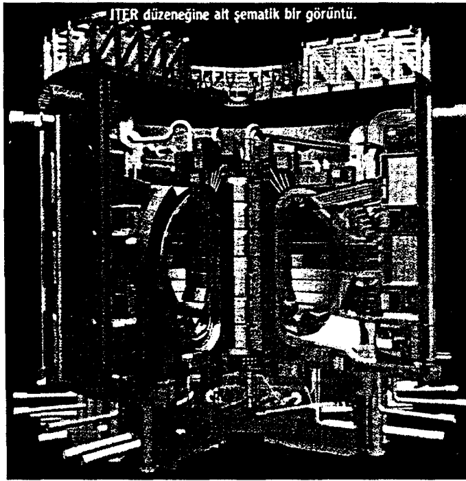
Şekil 5.4. ITER düzeneğine ait şematik bir görüntü [19]
