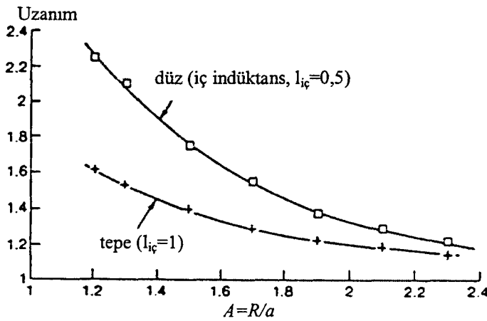
Şekil 6.4. Düzgün bir dikey alanda, tepe ( I_{iç}=1 ) ve düz ( I_{iç}=0,5 ) akım profilleri için uzanımın görünüm oranı ile değişimi [25]
