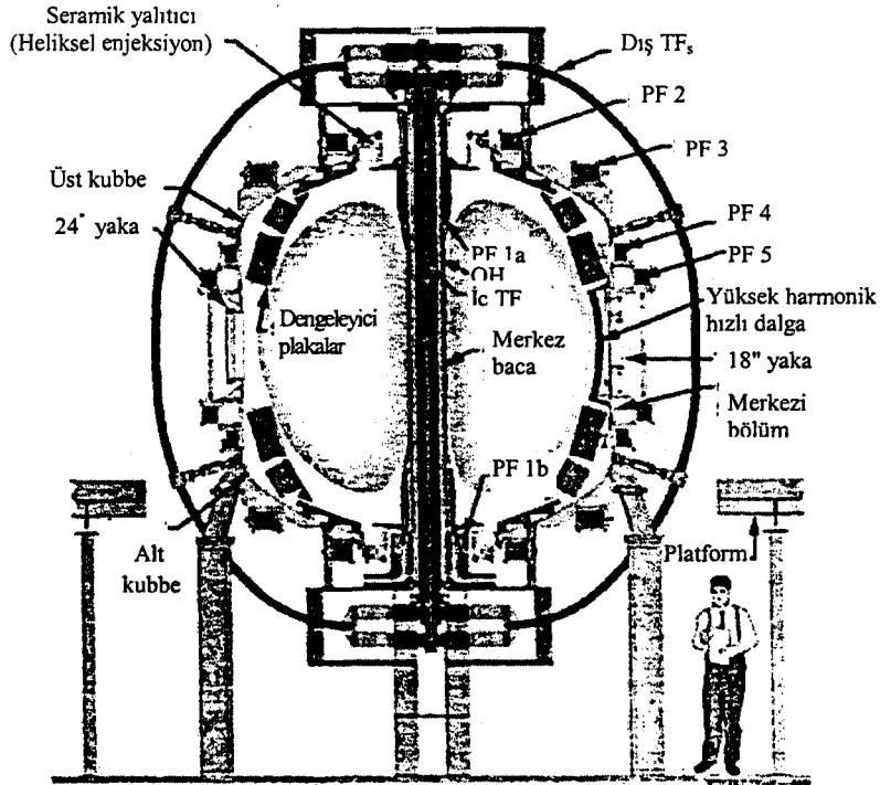
Şekil 7.15. NSTK aletinin iç yapısı [30]
