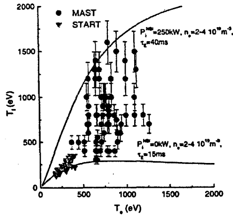
Şekil 7.11. İlk denemeler boyunca NBI ile ısıtılan boşalmalar için merkezî T_e (Thomson saçılmasından) ve T_i (NPA ölçümlerinden sonuçlanan) sıcaklıklarının çizimi. Eğri çizgiler, basit termal güç denge modelinin maksimum ve minimum tahminlerini gösterir [29]
