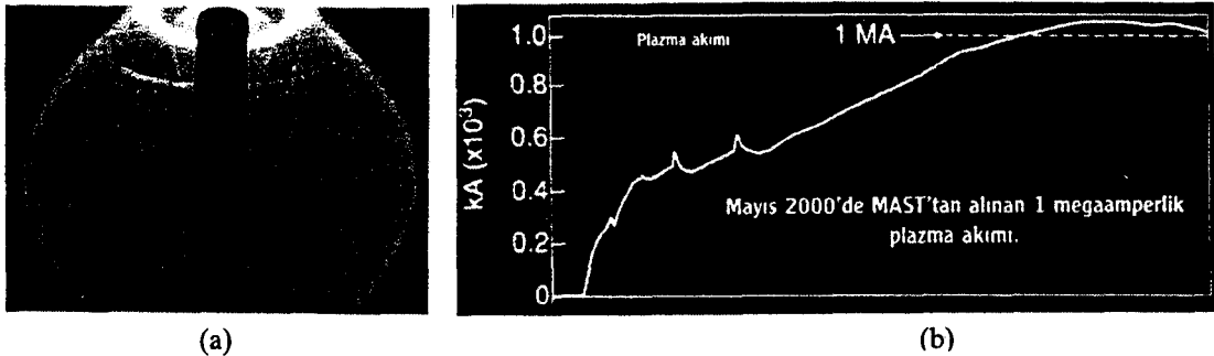
Şekil 7.13. (a) Hızlı fotoğraf tekniğiyle saptanmış 1MA'lık tokamak şekillenmesi (b) MAST'tan elde edilen 1MA'lık plazma akımı [19]
