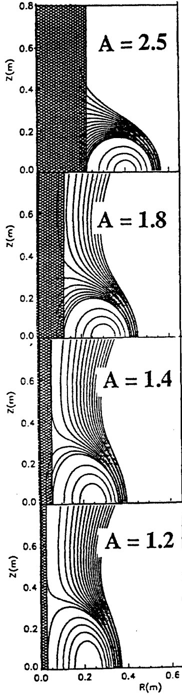
Şekil 6.3. Görünüm oranı 2,5, 1,8, 1,4 ve 1,2'de serbest-sınır denge karşılaştırması [25]
