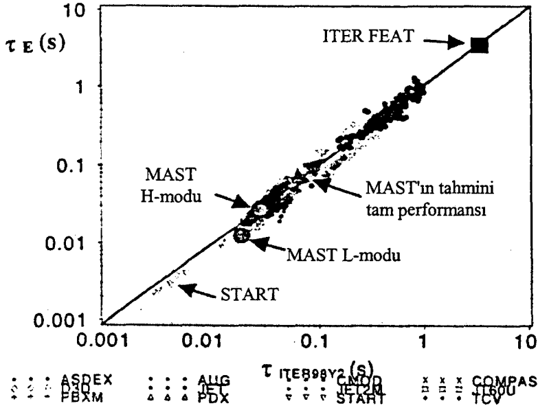
Şekil 7.12. ITER98PBY2 ölçeği ile karşılaştırılmış dünya tokamak ELMy H -mod kuşatma verileri [29]
