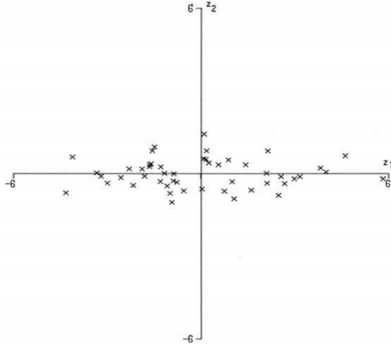
Şekil 3.2 Şekil 3.1 de gösterilen veri kümesinin temel bileşenler eksenindeki ( z_1 ve z_2 ) gösterimi.
