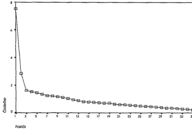
Şekil 2. Scree Sınaması
