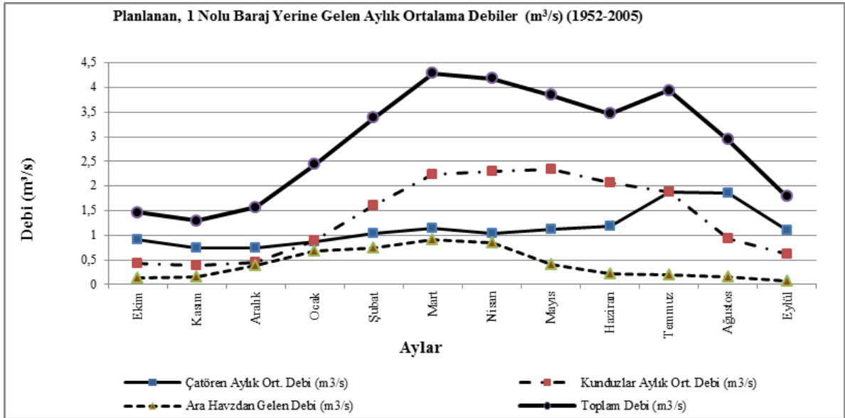
Şekil 13. Baraj gölüne giriş debileri (m 3 /s)
