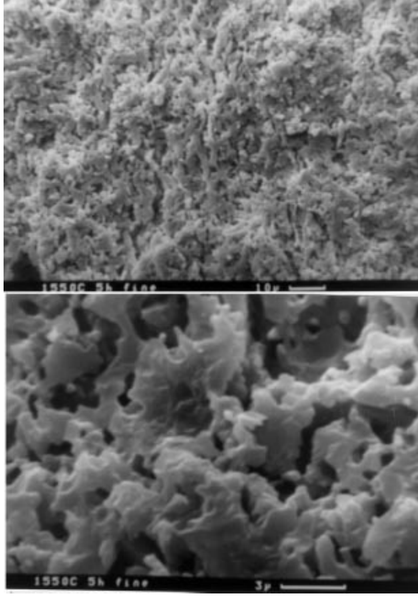
Şekil 6. İnce tozla hazırlanmış numunenin Taramalı Elektron Mikroskopi (SEM)'den alınan görüntüleri (Üstte 1000, altta 6000 büyütmede)
