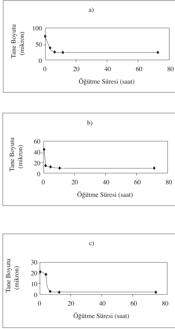
Şekil 1. \alpha -alüminanın öğütme süresiyle tane boyutu arasındaki bağıntı
