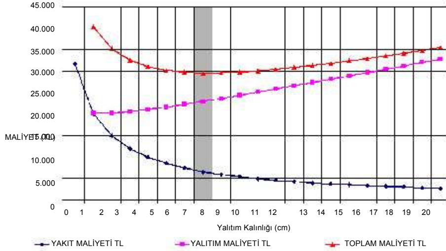
Şekil 7. Lojman Bloğu duvarlarında EPS kullanımına göre optimum ısı yalıtım kalınlıkları
