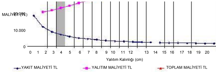
Şekil 9. Lojman Bloğu duvarlarında taş yünü kullanımına göre optimum ısı yalıtım kalınlıkları
