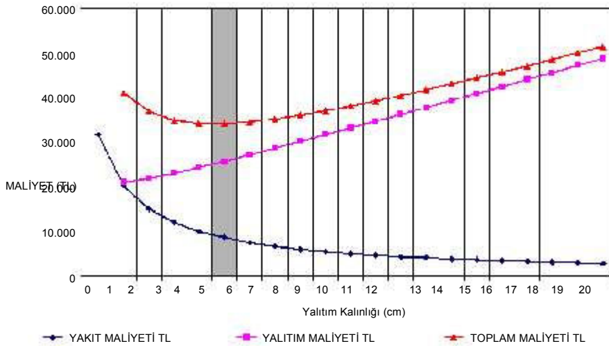
Şekil 8. Lojman Bloğu duvarlarında XPS kullanımına göre optimum ısı yalıtım kalınlıkları
