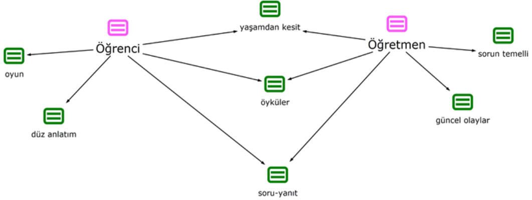
Şekil 3. Öğrenme-Öğretme Süreci
