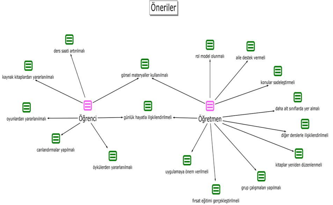
Şekil 7. Öneriler
