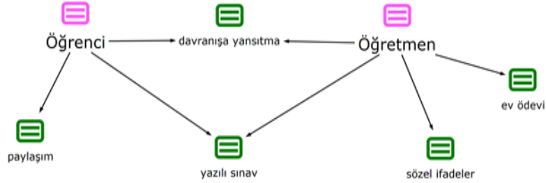
Şekil 5. Değerlendirme
