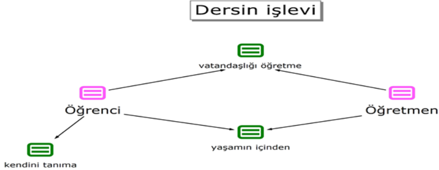
Şekil 1. Dersin işlevi
