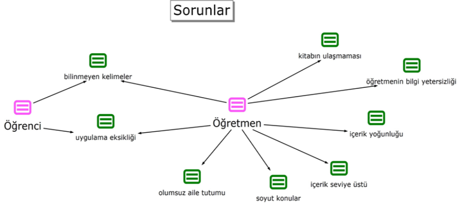
Şekil 6. Yaşanan sorunlar
