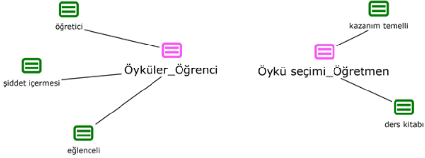
Şekil 4. Öyküler-öykü seçimi
