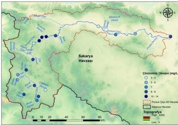
Şekil 2. pH, iletkenlik, çözünmüş oksijen ve bulanıklık parametreleri dağılım haritaları Figure 2. Distribution maps of pH, conductivity, dissolved oxygen and turbidity parameters
